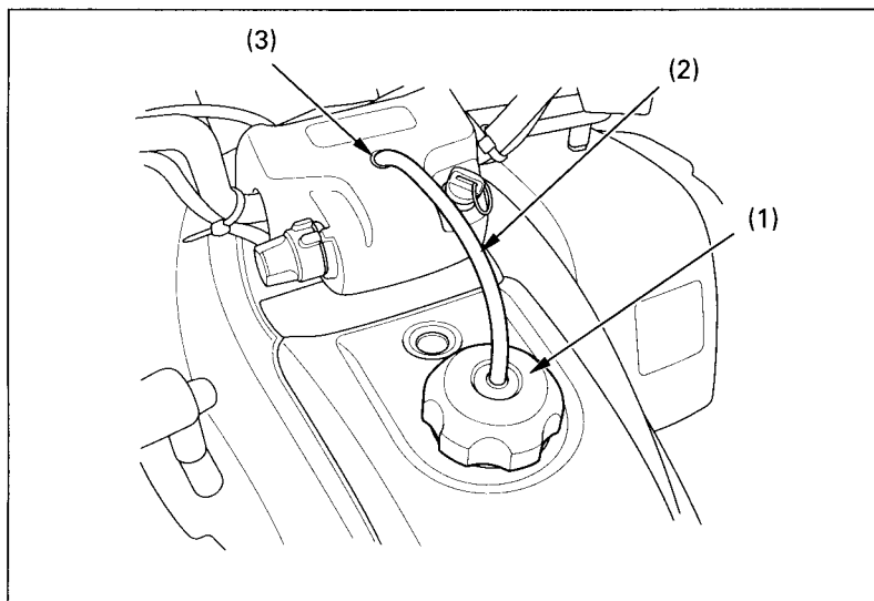
Fig. 2-29 (1) Fuel fill cap
