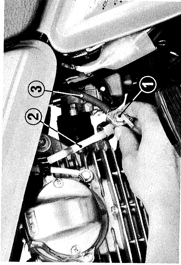
①フューエルコック ②フューエルストレーナ ③フューエルチューブ
