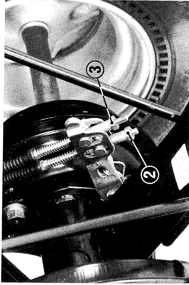
②ペダルアジャスタ ③レバーアジャスタ
