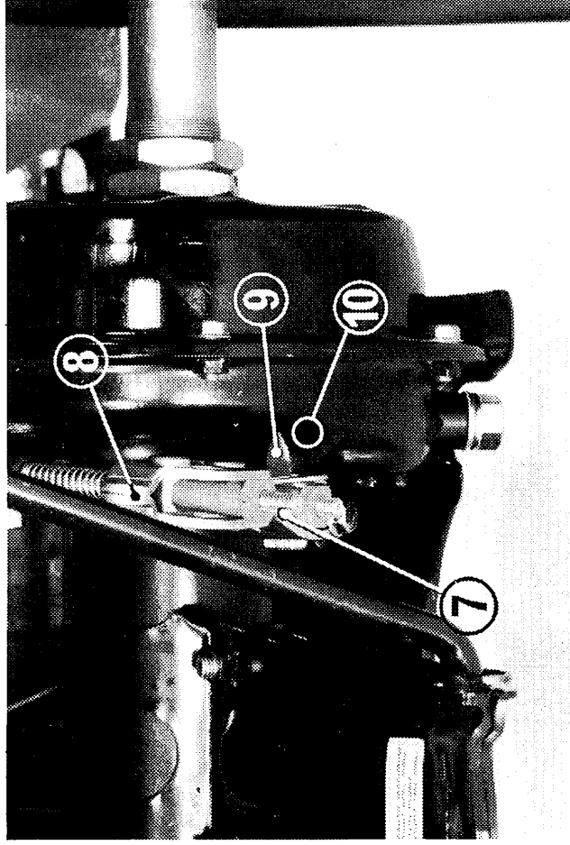
⑦ロアーアジャスタ ⑧ブレーキアーム ⑨矢印
