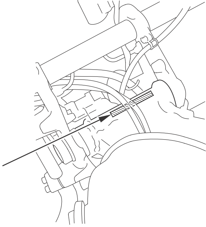
フレーム号機打刻位置
