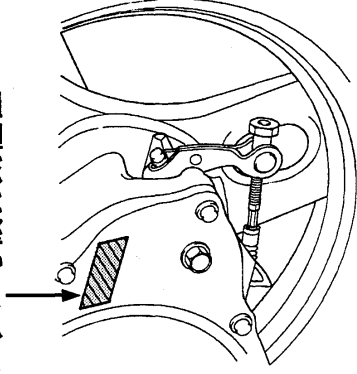
エンジン号機打刻位置
