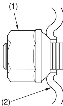
(2) wheel rim
